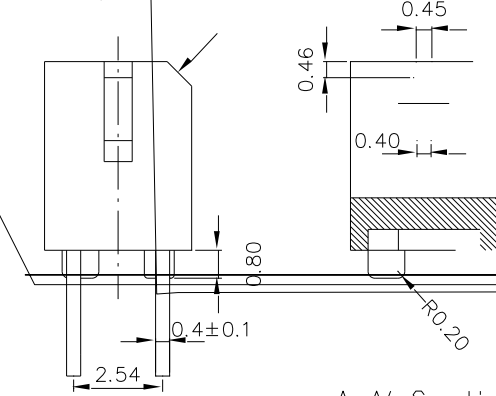
A-A' Section
